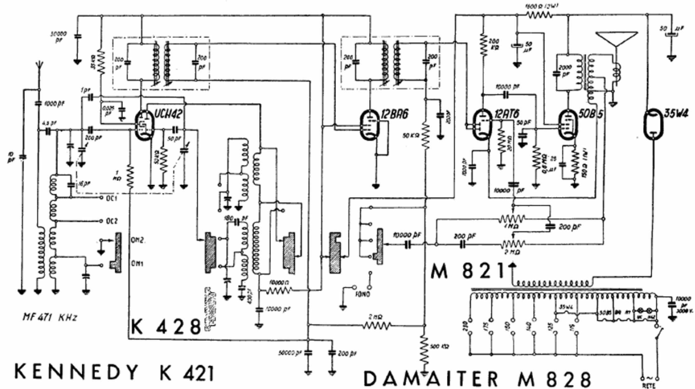
MAGNADYNE RADIO - Mod. Damaiter M 828, mod. Kennedy K 421 e mod. Damaiter M 821. Onde medie suddivise e due gamme di onde corte. Media frequenza 471 kc/s. Controllo di volume con compensazione variabile dei toni bassi, a reazione inversa. I filamenti delle valvole sono collegati a più prese del primario del trasformatore di alimentazione (i modd. Kennedy K 421 e Damaiter M 828 sono sprovvisti di presa per pick-up).
